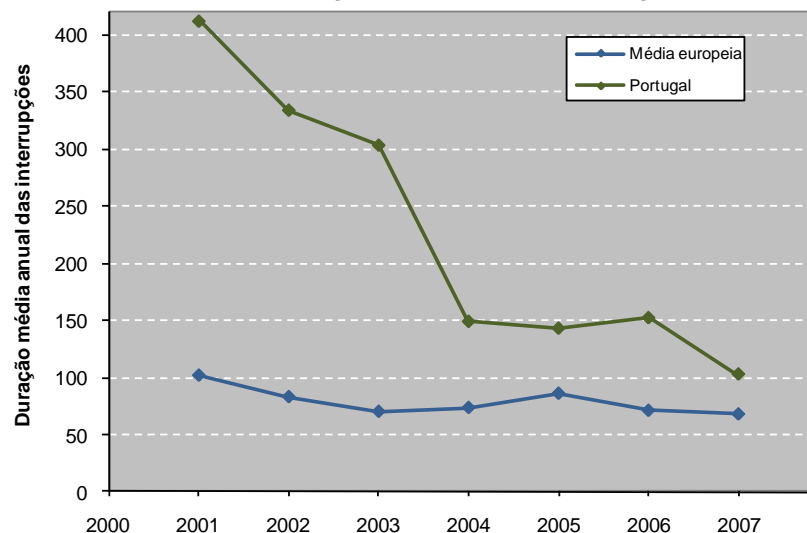
Duração das interrupções
