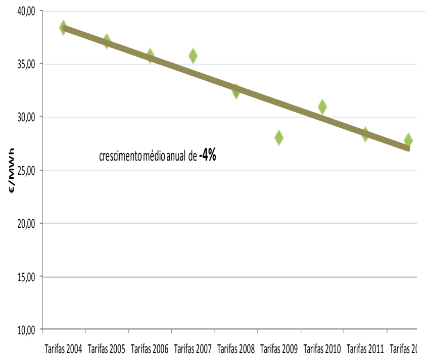
Evolução dos custos com as redes (€/MWh)
